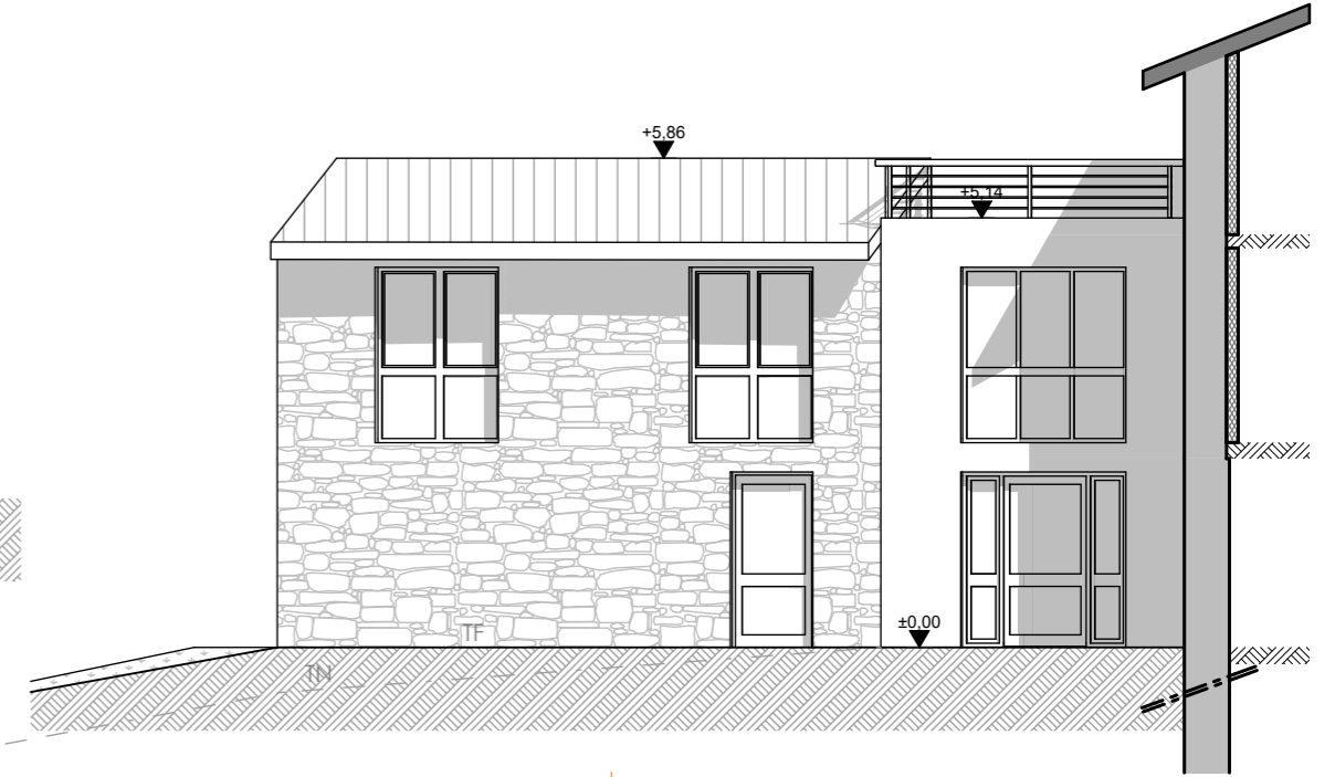
Façade OUEST
