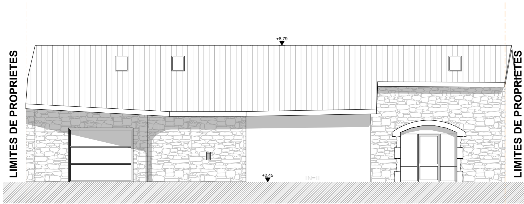
Façade NORD
